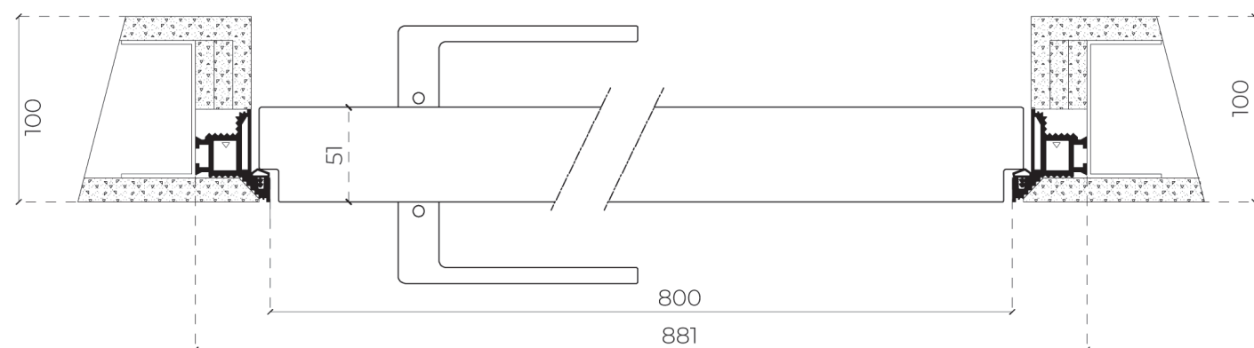
RASO MURO CIECA | DX A SPINGERE
