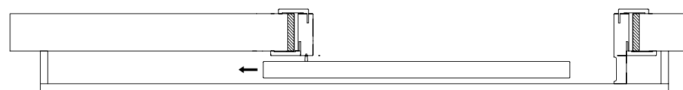
PORTA SCORREVOLE ESTERNO MURO CON MANTOVANA SPINTA A SINISTRA
